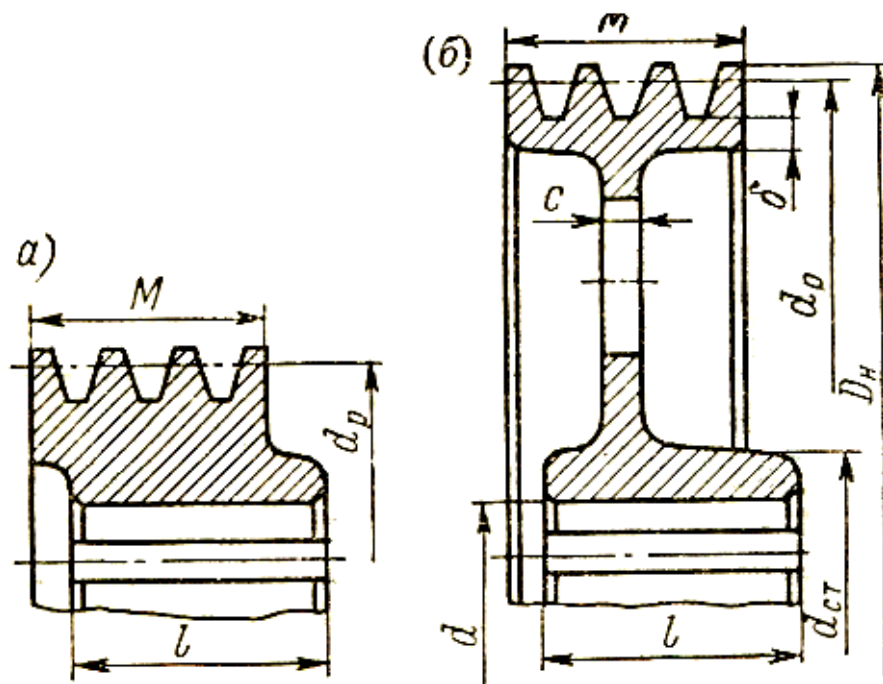
Рис.7.3 Шкивы для клиновых ремней:
