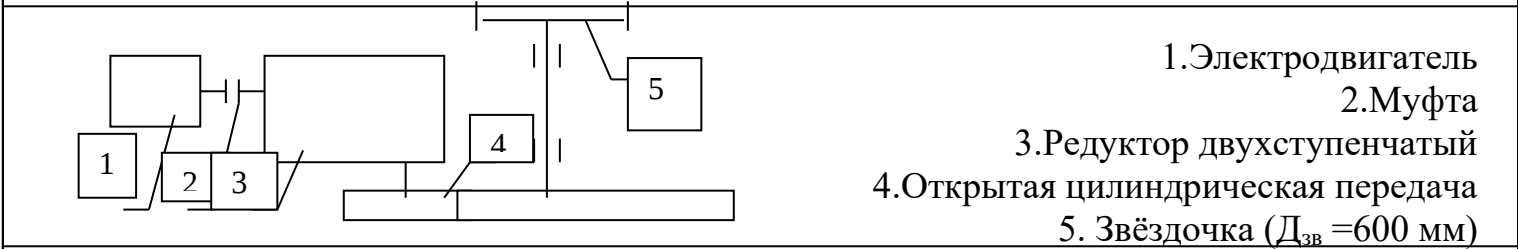
Схемы редукторов.
